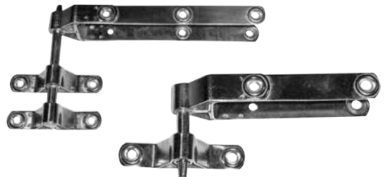
SR20538 Krom İğnecik No:1 Aynakıç Takım SR20540 Krom İğnecik No:1 Bodoslama Takım • 304 Kalite
