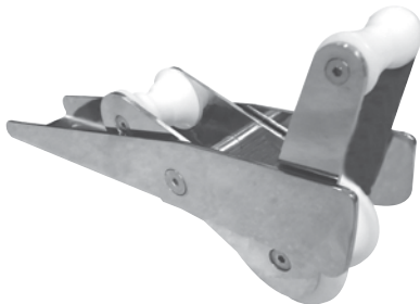
SR20232 Mafsallı Burun Makarası 75 x 400 mm SR20233 Mafsallı Burun Makarası 75 x 500 mm SR20235 Mafsallı Burun Makarası 110 x 600 mm SR20236 Mafsallı Burun Makarası 110 x 700 mm Not: Delta Çapalara Uygundur • 316 Kalite
