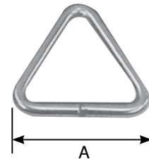
SR23170 Krom Üçgen 04 mm - A: 40x40 mm SR23172 Krom Üçgen 05 mm - A: 50x50 mm SR23174 Krom Üçgen 06 mm - A: 60x60 mm SR23176 Krom Üçgen 08 mm - A: 76x76 mm SR23178 Krom Üçgen 10 mm - A: 99x99 mm • 304 Kalite
